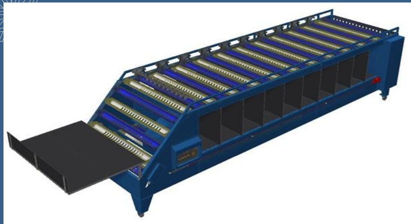
Jamafa Länge sortiermaschine mit Doppelfunktion mit 1 Auflagetisch
